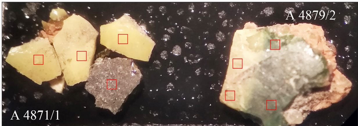
Рис. 3. Фіксація елементного складу на зразках в ході спектрального аналізу Fig. 3. Fixation of elemental composition on samples during spectral analysis
