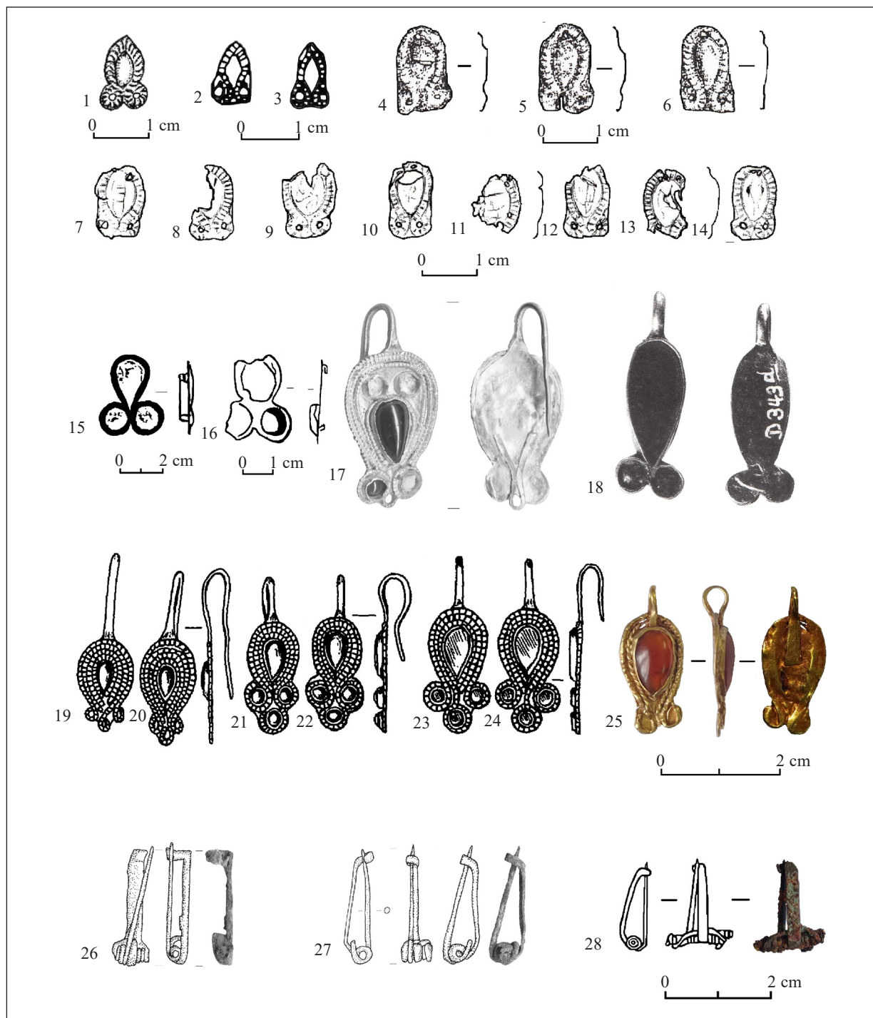
Рис. 12. Речі з кургану № 17 (25, 28) та аналогії (1–24, 26–27): 1 — курган № 1, Нагорное (за: Гудкова, Фокеев 1984, с. 40, рис. 1: 2); 2–3 — поховання 38, некрополь Ніконія (за: Бруйко, Дзиговський, Секерская 2008, с. 157, рис. 75: 11); 4–6 — могила № 49, Дружное (за: Храпунов 2002, с. 234, рис. 134: 26); 7–14 — могила № 110, Нейзац (за: ред. Храпунов 2011, с. 113, рис. 49: 54–61); 15 — поховання 4, Лермонтівська Скеля 1 (за: Мастыкова 2009, с. 261, рис. 10: 1); 16 — Свободний Аул (за: Абрамова 1997, с. 74, рис. 49: 17); 17 — могила 65, Алмалик (за: Mączyńska et al. 2016, Taf. 37: 4); 18 — Майкоп (за: Мастыкова 2009, с. 358, табл. 62: 3); 19–24 — могила 82, склепи 88, 126 могильника Лучісте (за: Айбабин, Хайредінова 2008, с. 49, рис. 26: 3–5); 26–27 — могила 65, Алмалик (за: Mączyńska et al. 2016, Taf. 34: 3.1–3.2)
